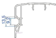
Marco doble riel 100SN1090
