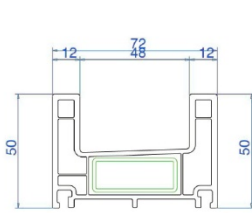
Marco doble riel 100SN1090
