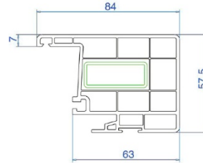
Travesaño 100SN3001
