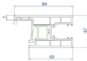
Hoja Ventana 100SN2001
