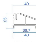
Cubierta marco monorriel 100SU6050
